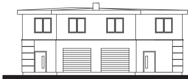
ELEWACJA ZACHODNIA 1:100
